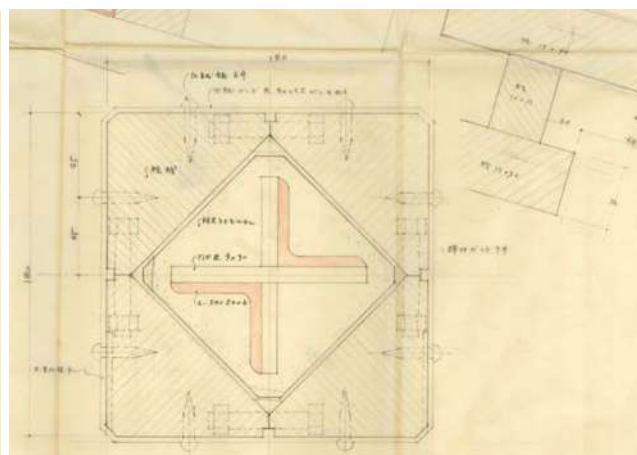
複合柱原寸図（提供：高知県）
