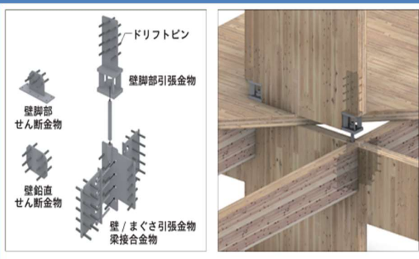
【CLT パネル接合金物】
